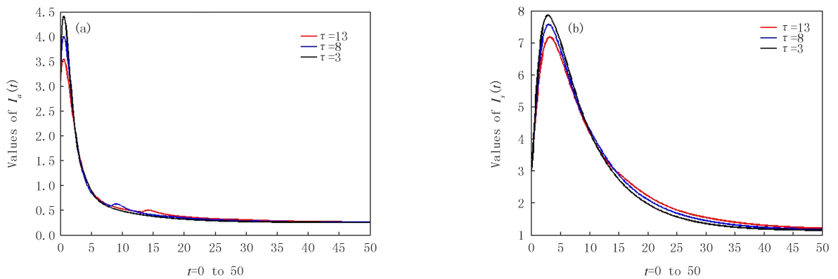
图2 R_0 > 1 时, I_a(t) (a) 与 I_s(t) (b) 在不同时滞下的趋势图 Fig.2 When R_0 > 1 , trend diagram of I_a(t) (a) and I_s(t) (b) with different time delays
