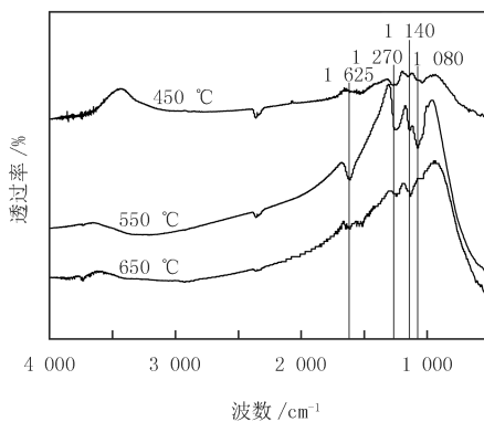
图 1 样品分别于 450 、 550 、 650\text{ }^\circ\text{C} 煅烧后的红外光谱图
