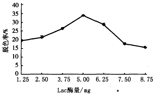
图 5 Lac酶量对氨基黑10B脱色的影响
