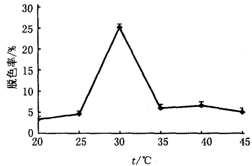
图 2 温度对氨基黑10B脱色的影响
