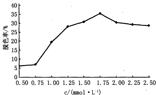
图 3 硫酸铜对氨基黑10B脱色的影响
