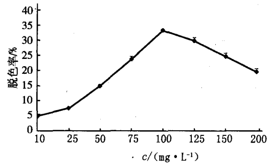
图 6 氨基黑浓度对氨基黑10B脱色的影响
