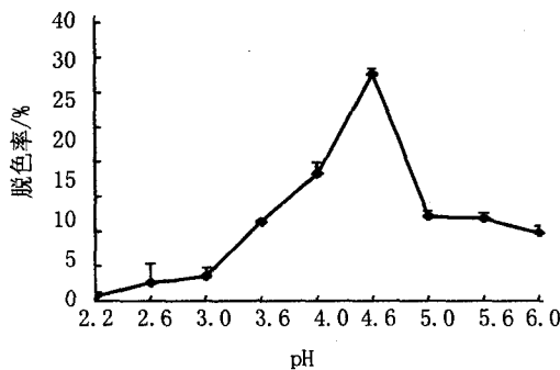
图 1 pH对氨基黑10B脱色的影响
