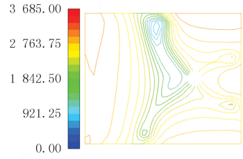
图4 传热系数分布[W/(m 2 ·℃)]
