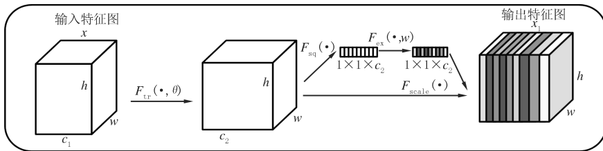
图3 SENet模块
