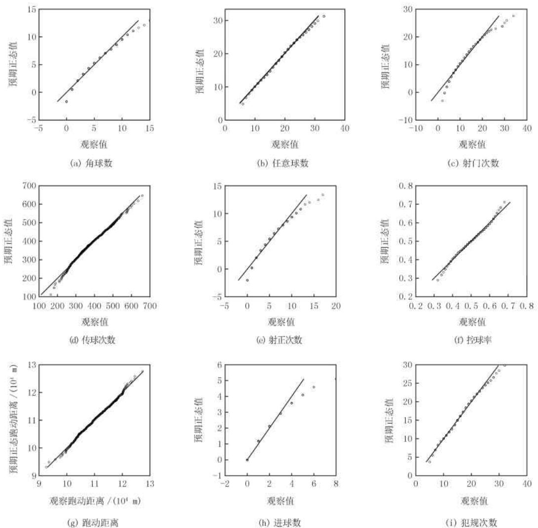
图1 各项统计 q-q 图
