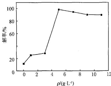
图6 Fe 3 O 4 /α-Fe 2 O 3 的投加量对亚甲基蓝降解率的影响
