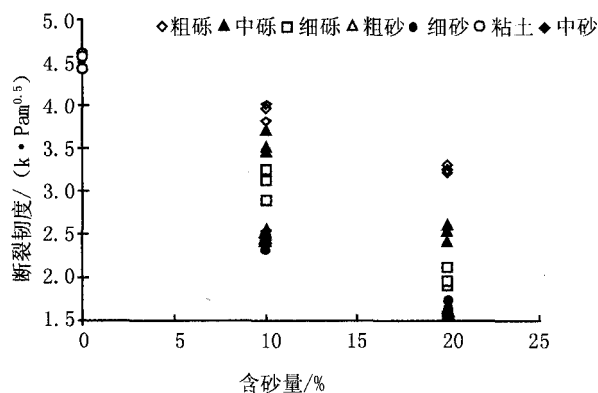
图5 含砂量与断裂韧度关系曲线
