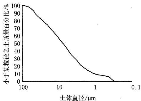
图3 试验土料颗粒级配曲线
