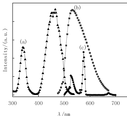
(a) Ce 3+ 单掺样品(YAG:1.0% Ce 3+ )中 Ce 3+ 的激发光谱(λ em =531 nm);(b) Ce 3+ 的发射光谱(λ ex =460 nm);(c) Nd 3+ 单掺样品(YAG:1.0% Nd 3+ )中 Nd 3+ 的激发光谱(λ em =1 064 nm).
