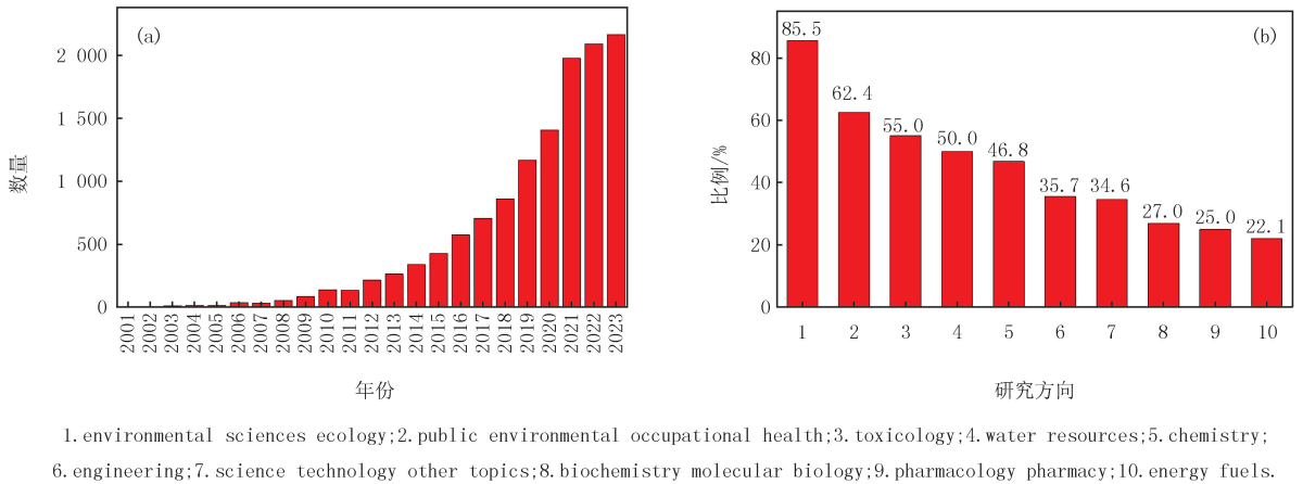
图1 WOS数据库中2001至2023年关于新污染物的论文
