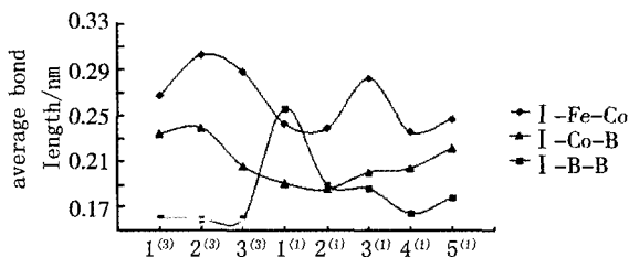
图5 团簇Co 2 FeB 2 中各稳定构型的平均键长
