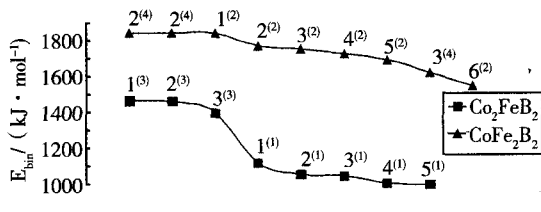
图2 团簇 Co_2FeB_2 , CoFe_2B_2 各构型结合能
