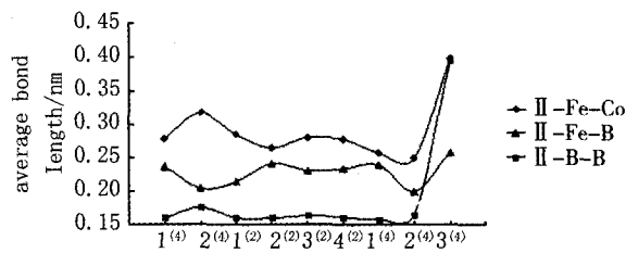
图6 团簇CoFe 2 B 2 中各稳定构型的平均键长
