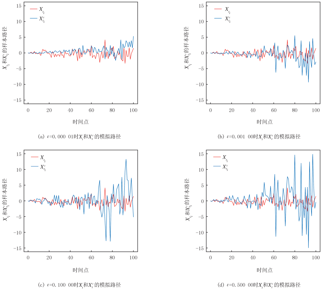
图2 X_t 和 X_t^\epsilon 的模拟样本路径
