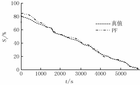
图4 S_0=80\% 的追踪仿真图
