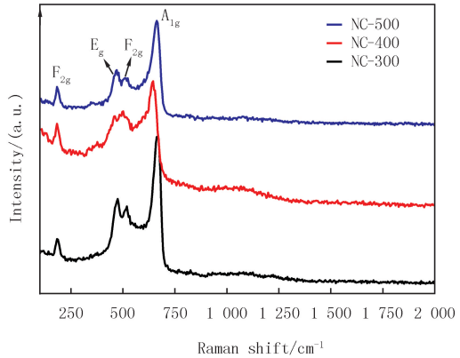
图4 OER反应前样品的拉曼光谱图
