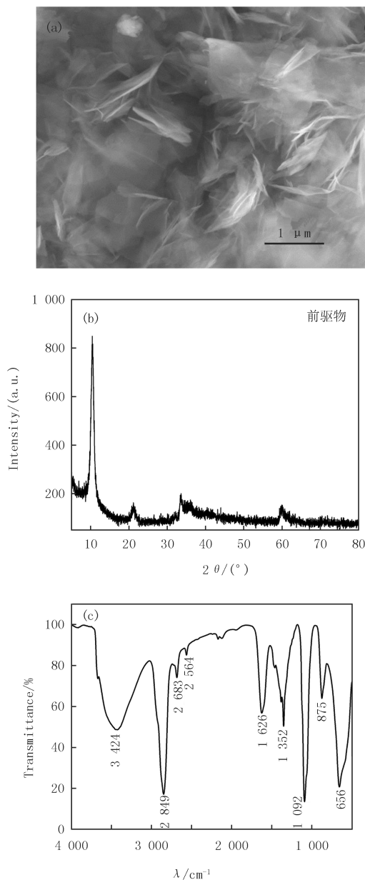
图1 溶剂热前驱物的SEM照片(a), XRD图谱(b), 傅里叶红外吸收光谱(c)
