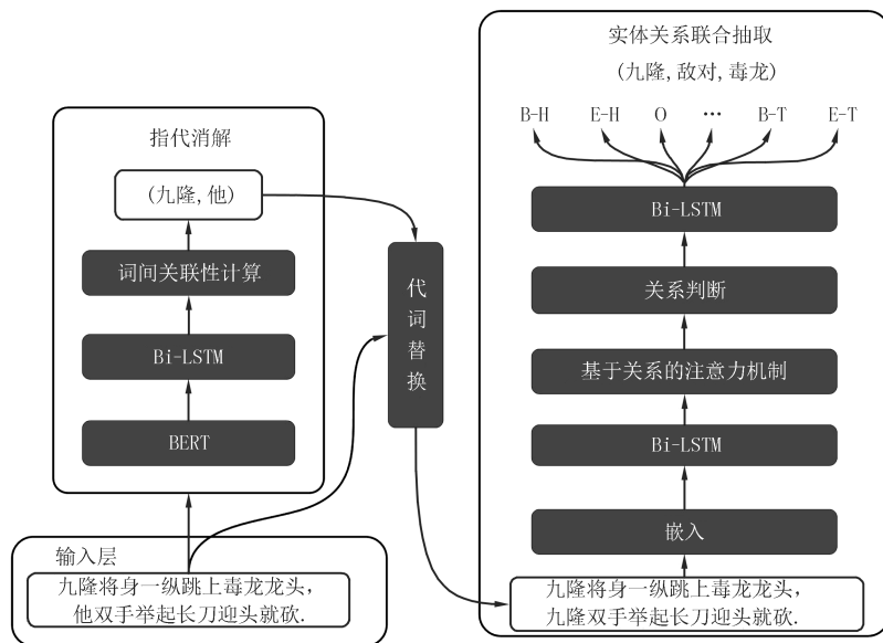
图1 模型架构图
