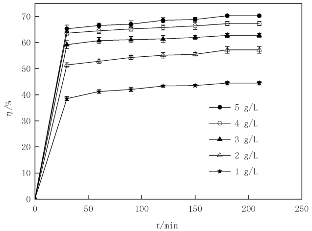
图9 投加量对MO去除率的影响
