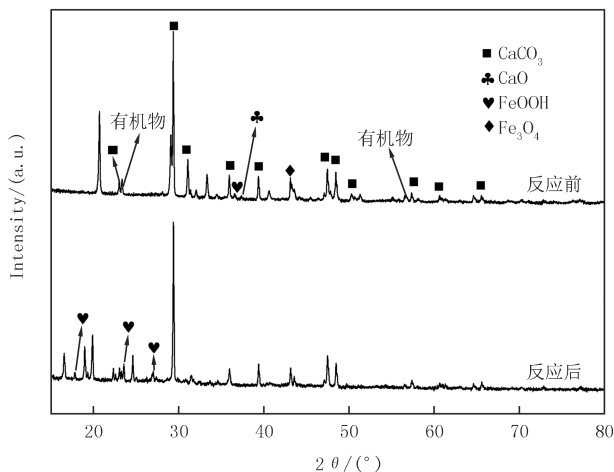
图7 与MO反应前后的TP-nZVI/S的XRD图谱
