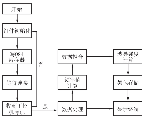
图7 单片机工作流程 Fig.7 MCU workflow
