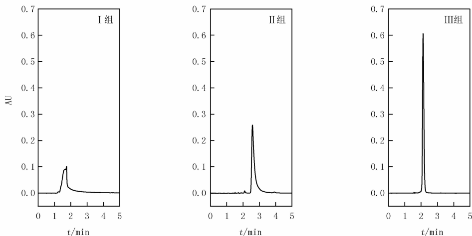
I 组: 甲醇和 0.1% 磷酸水溶液; II 组: 甲醇和高纯水; III 组: 甲醇和 0.02 mol · L -1 三乙胺水溶液.
