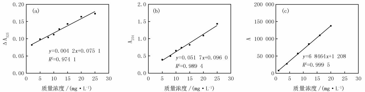
a. 褪色分光光度法; b. 紫外分光光度法; c. 高效液相色谱法.
