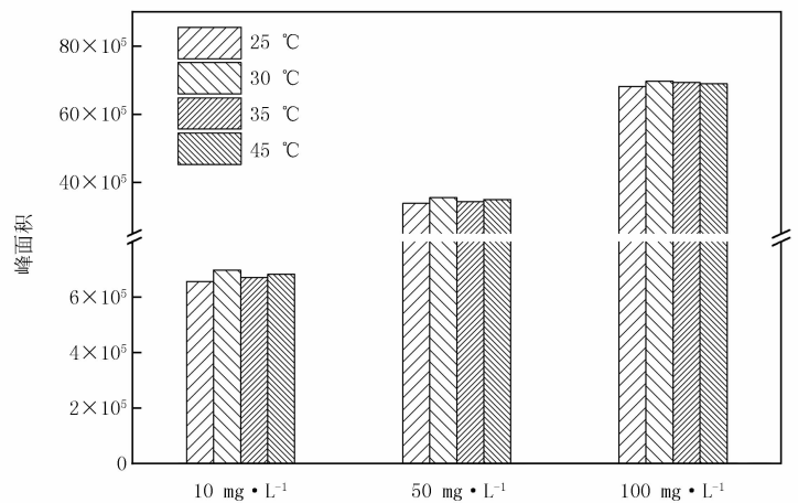
图2 不同温度条件下10、50和100 mg · L -1 头孢曲松钠的色谱峰面积比较
