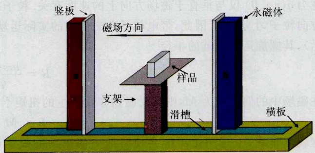
图3 磁场装置示意图
