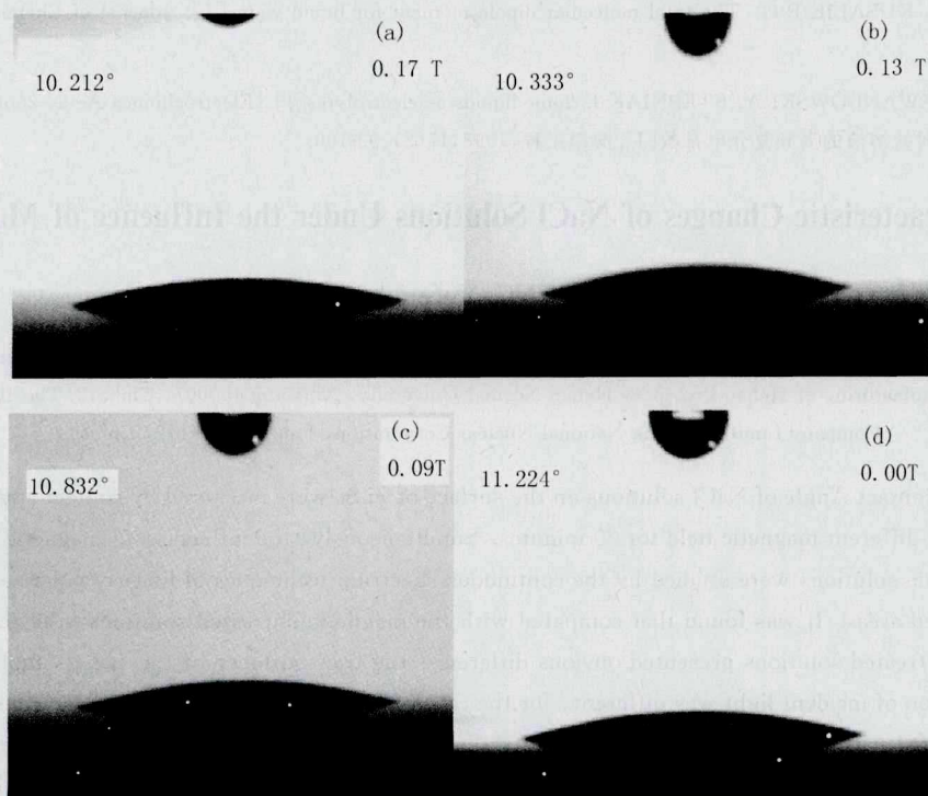
图6 经不同强度磁场处理后的浓度为1.5 mol/L的NaCl溶液在硒化锌表面的接触角
