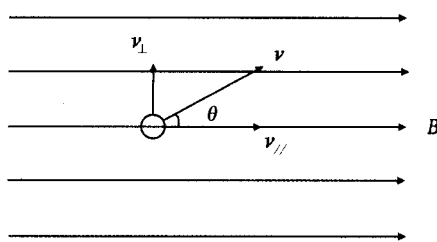
图1 粒子在磁场中的运动方向
