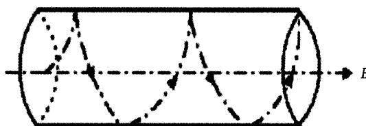
图2 粒子在磁场中的运动轨迹假设水分子
